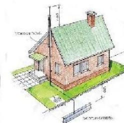
Устройство громоотвода
