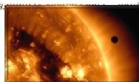
Атмосфера Венеры
