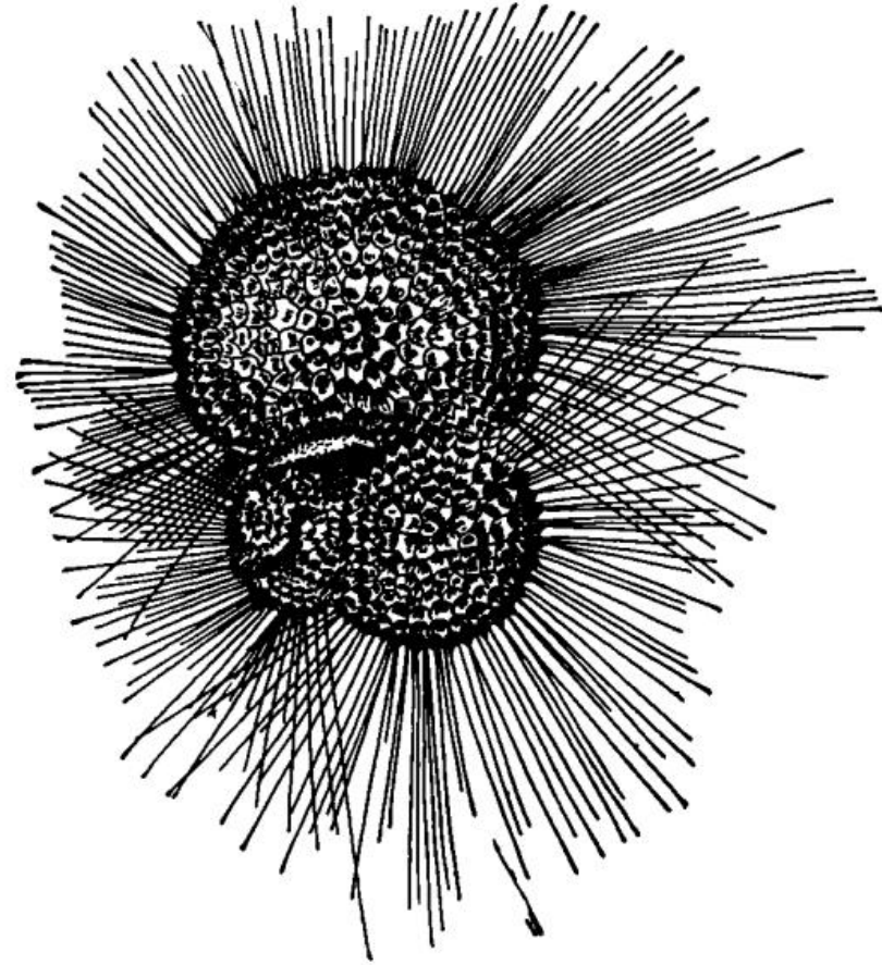
Рис. 36. Планктонная фораминифера Globigerina bulloides .
