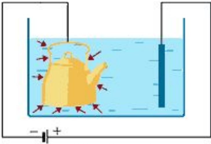
гальваностегия
