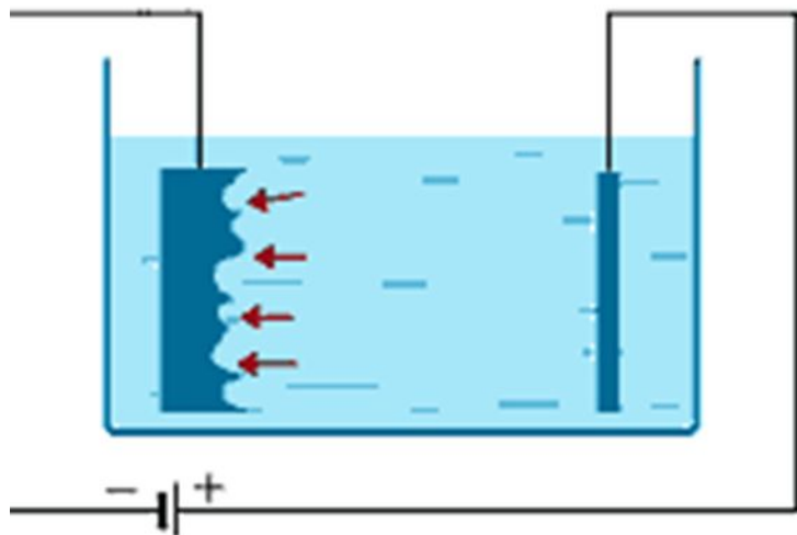
гальванопластика
