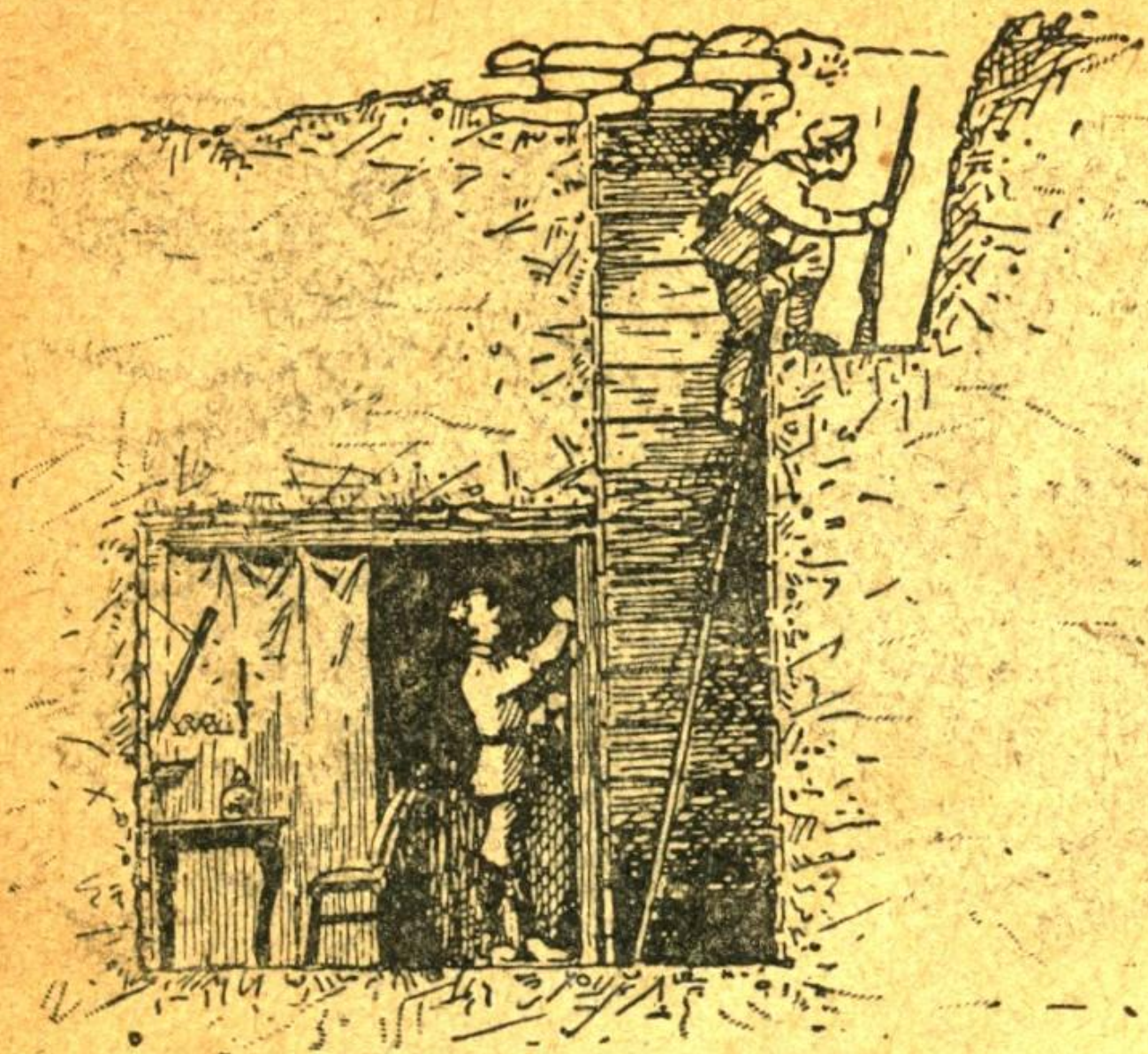
Профиль германскаго окопа съ помѣщеніемъ для отдыха и укрытія отъ огня.
