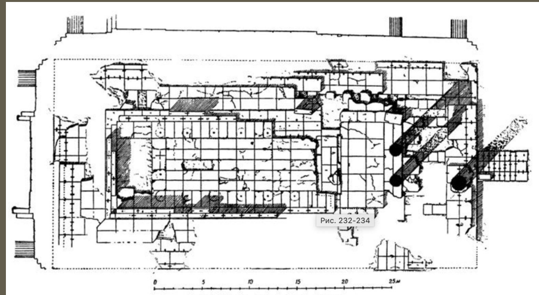
Храм Зевса. План
