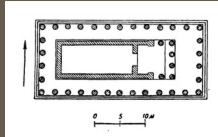
Реконструкция первоначального плана храма
