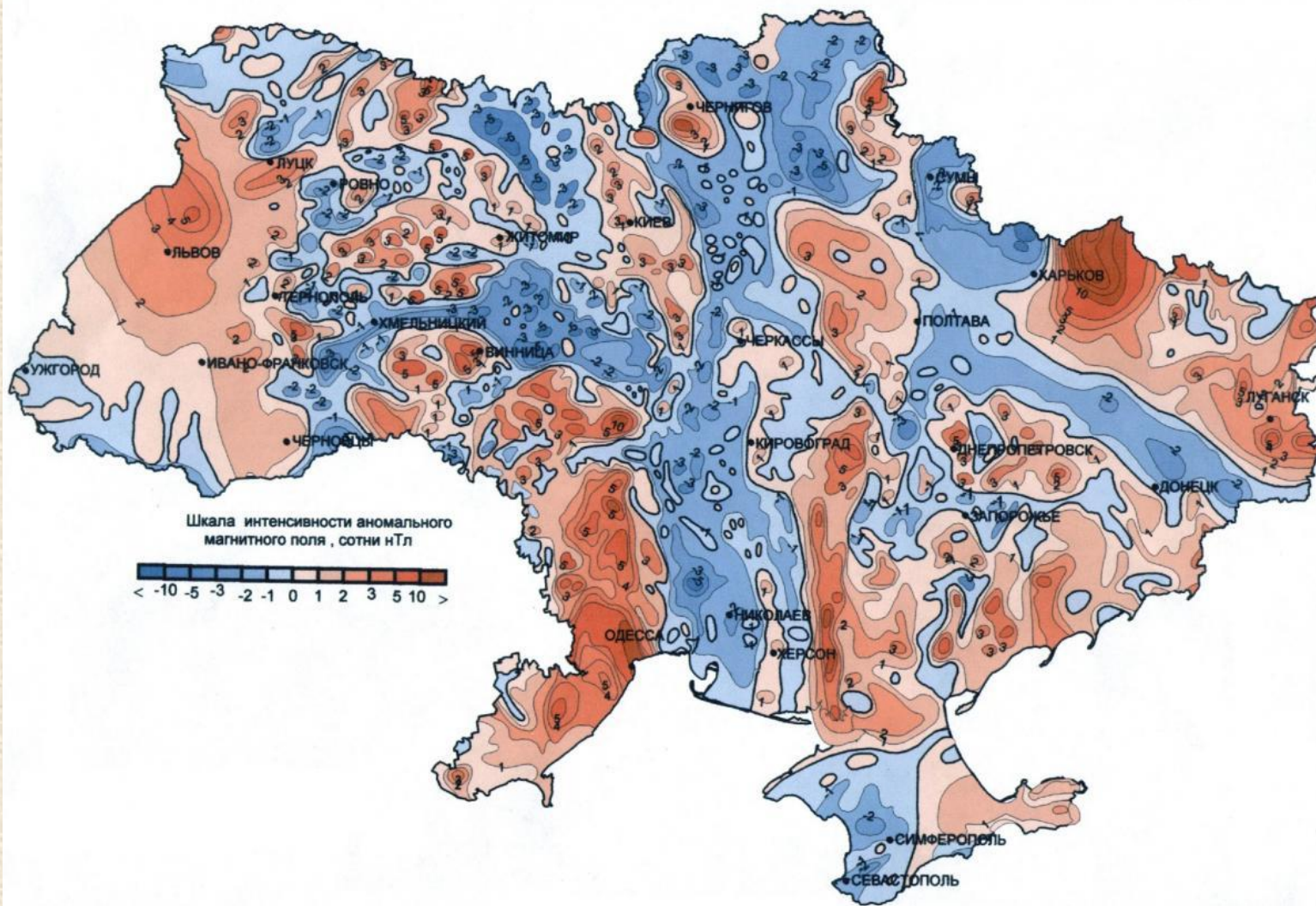
Карта аномального магнитного поля ( \Delta T_a ) Украины.
