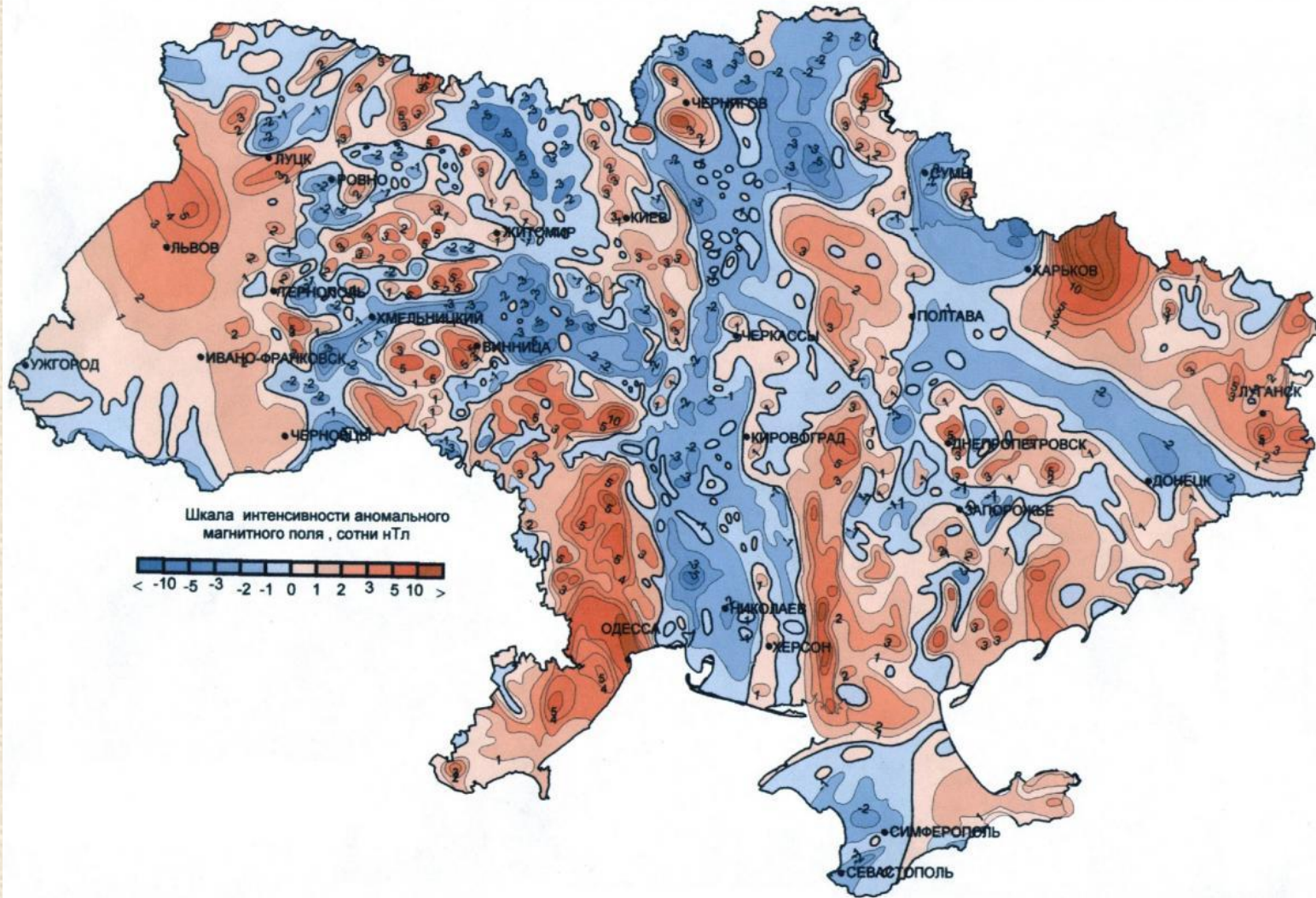
Карта аномального магнитного поля ( \Delta T_a ) Украины.
