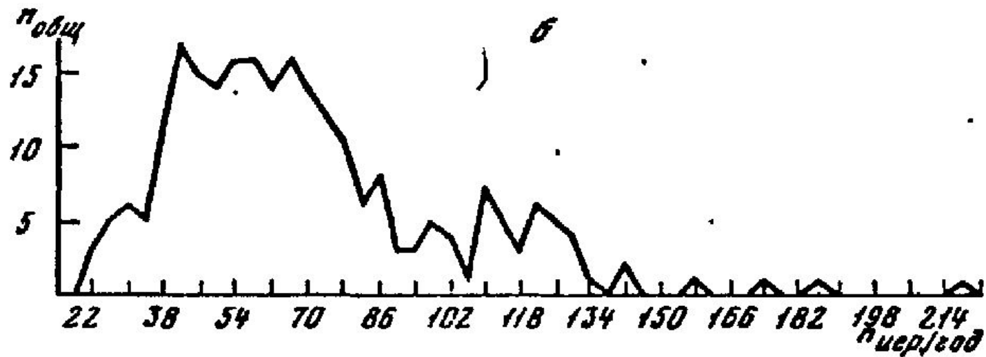
Рис. 1. Объем текста (а) и число иероглифов на 1 год (сгруппировано по 4 (б)).
