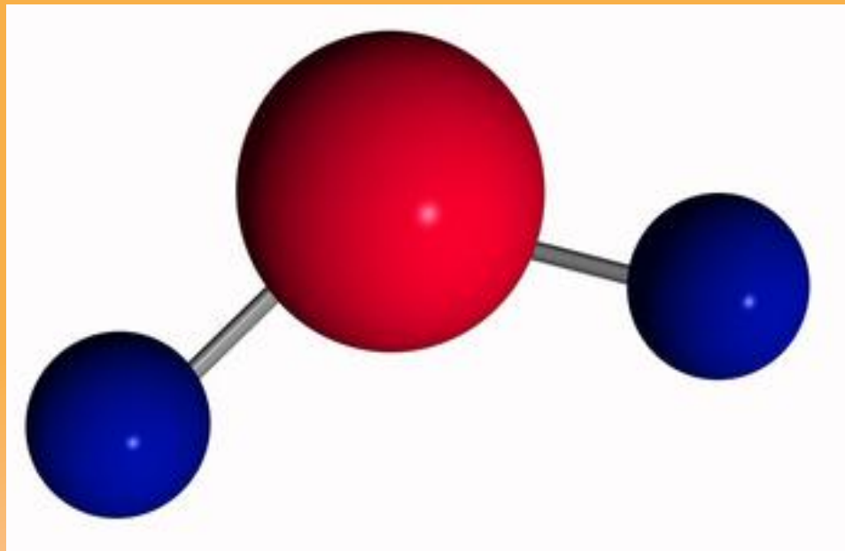
МОЛЕКУЛА ВОДЫ
