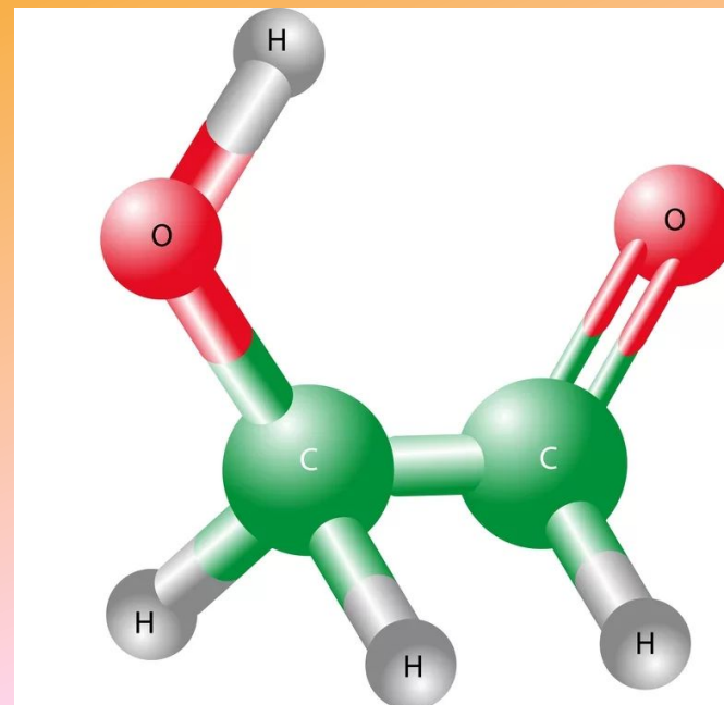
МОЛЕКУЛА САХАРА
