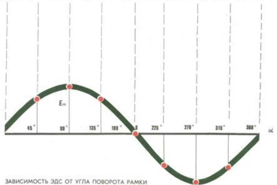
ЗАВИСИМОСТЬ ЭДС ОТ УГЛА ПОВОРОТА РАМКИ
