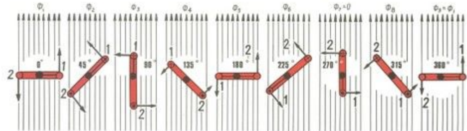
Положение рамки в магнитном поле
