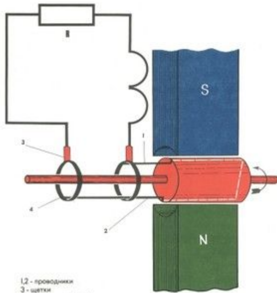
УСТРОЙСТВО ГЕНЕРАТОРА ПЕРЕМЕННОГО ТОКА
