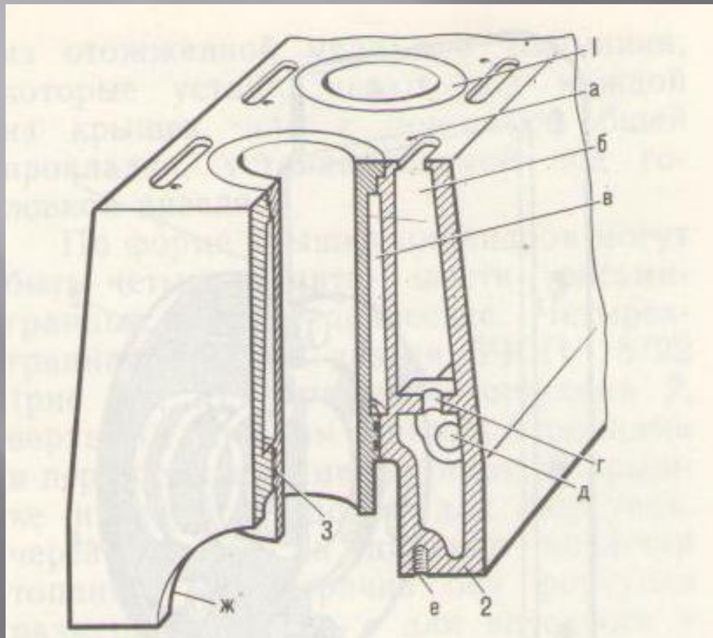
Блок цилиндров
