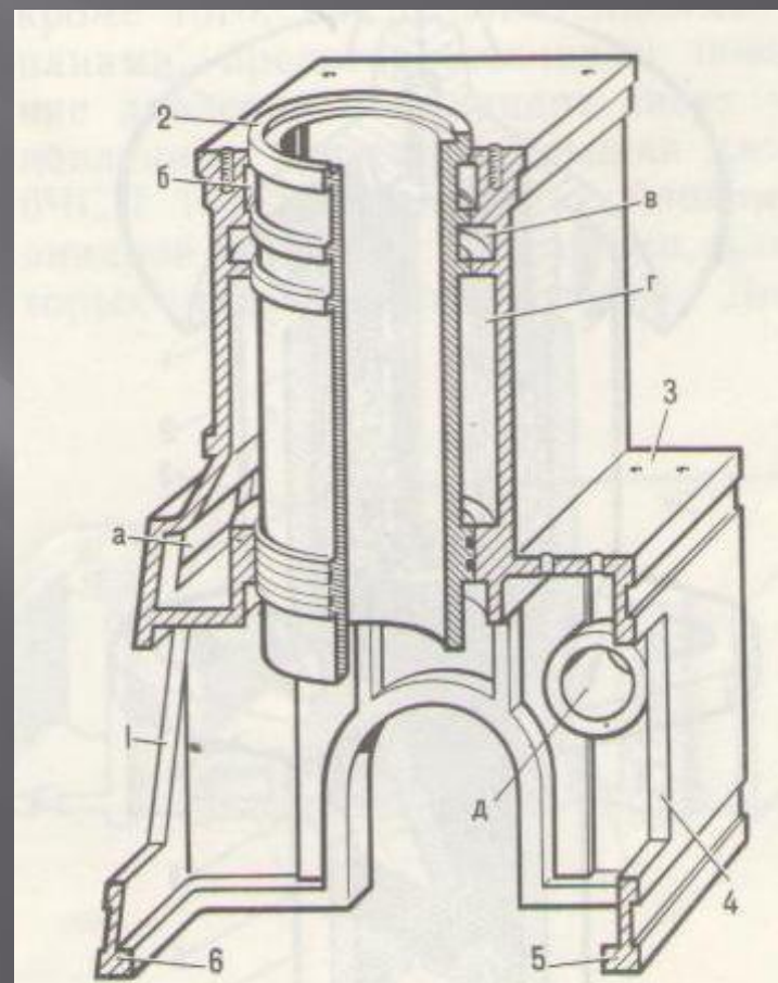
Блок-картер
