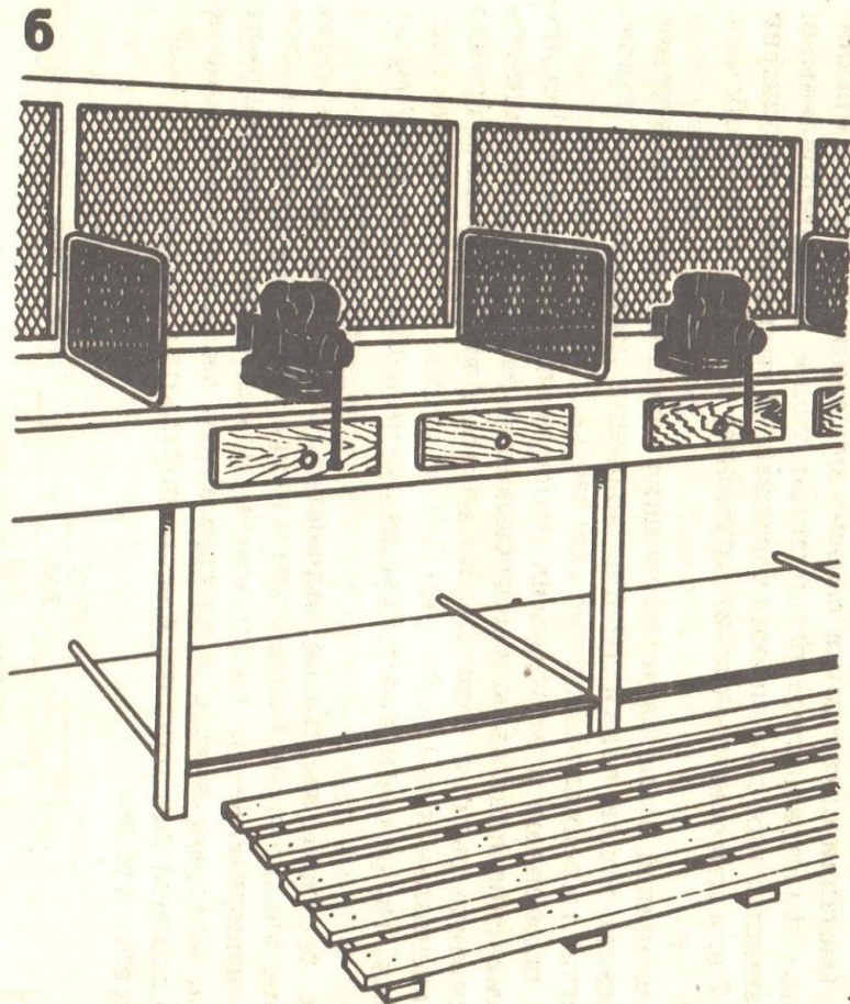
Рис. 1. Слесарные верстаки с поворотными тисками: а – одностольный, б – многостольный; 1 – каркас, 2 – столешница, 3 – тиски, 4 – защитный экран, 5 – планшет для чертежей, 6 – светильник, 7 – полочка для инструмента, 8 – планшет для рабочего инструмента, 9 – ящики, 10 – полки, 11 – сиденье
