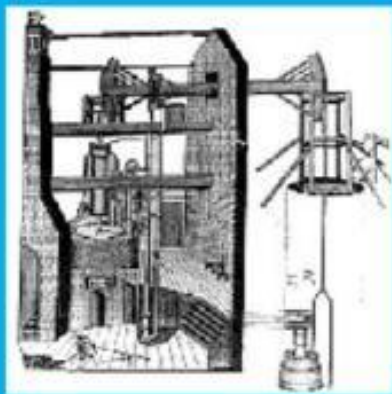
Первая паровая машина Ньюкомена
