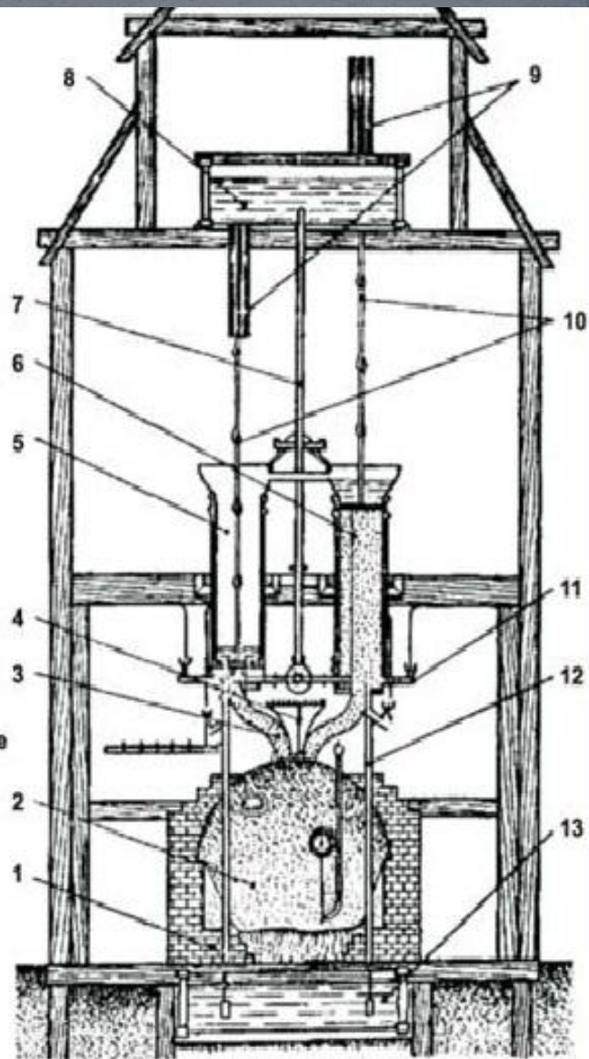
Схема устройства паровой машины И.И. Ползунова
