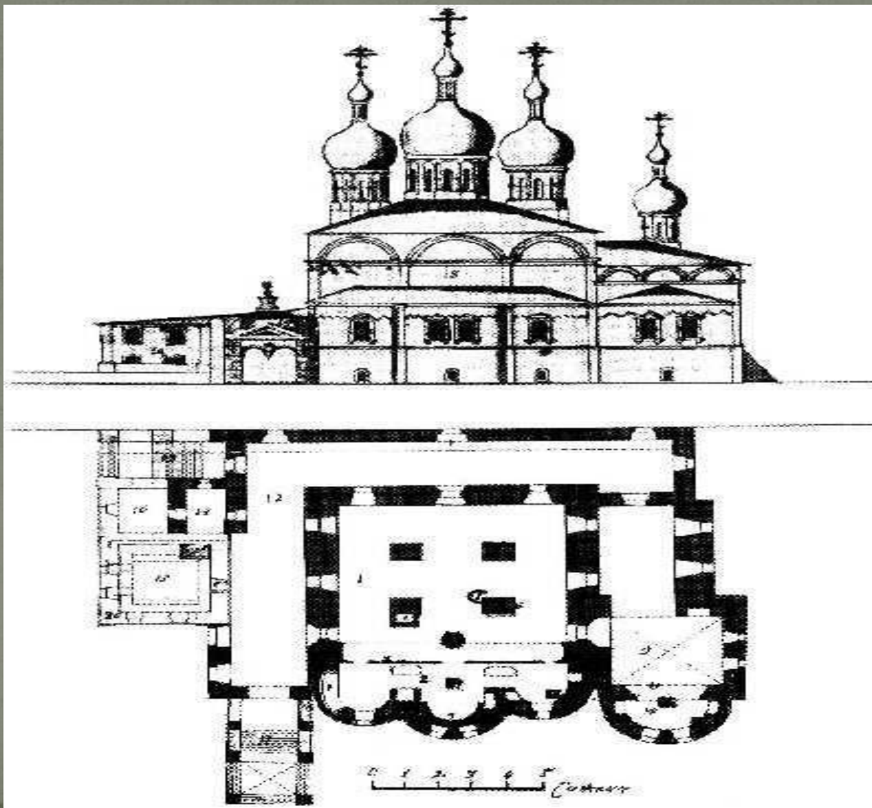
Успенский собор в XVI-XVII вв. Западный фасад и план. Чертёж 1773 г
