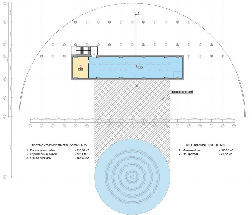
ПЛАН НА ОТМЕТКЕ -2,510
