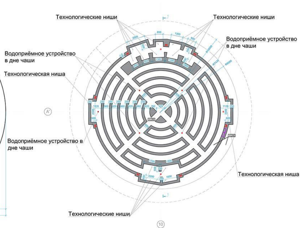
ПЛАН НА ОТМЕТКЕ -0,280
