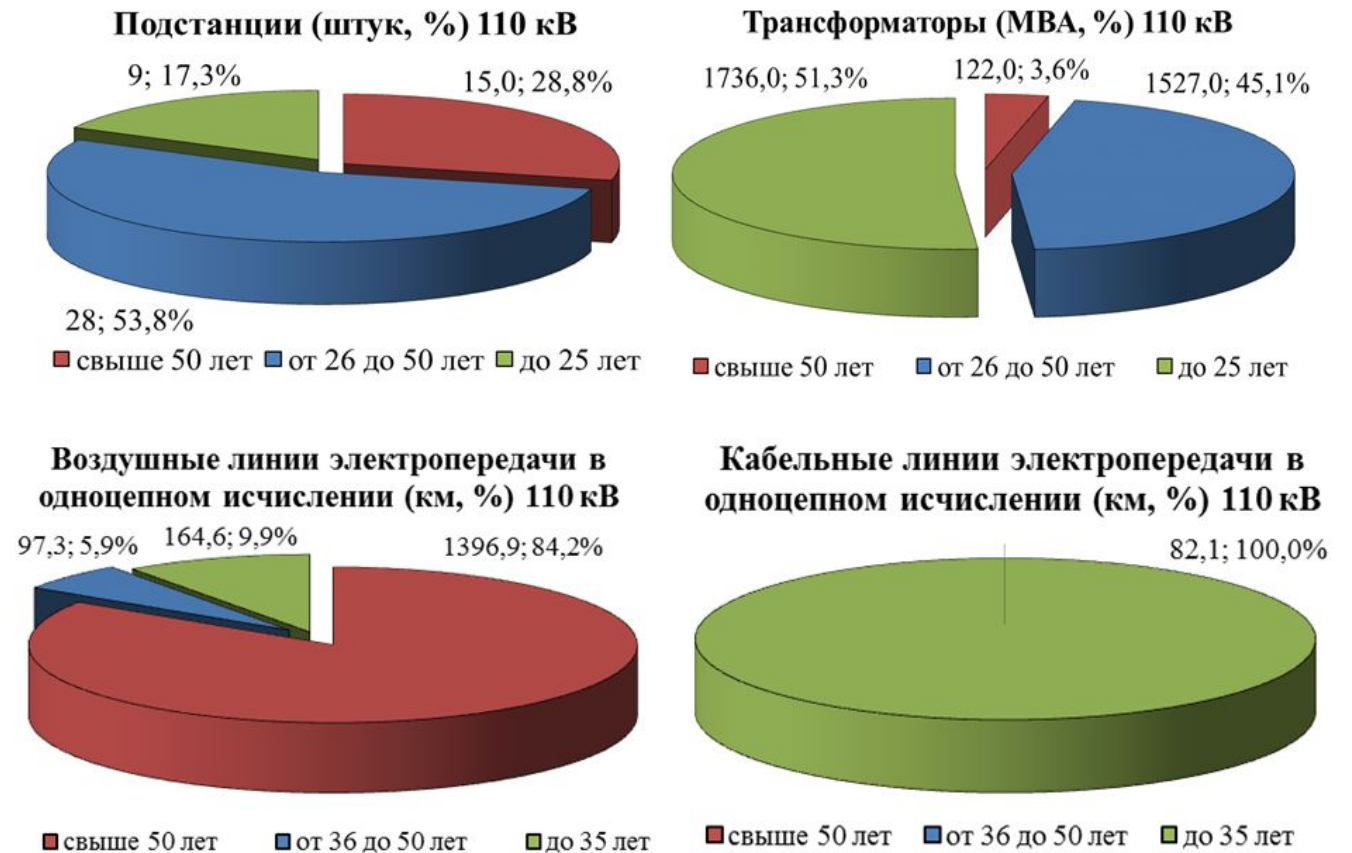
Рисунок 1.1 – Возрастная характеристика ВЛ, КЛ и ПС 110 кВ [сети предприятия 1] на 01.01.2019 г.
