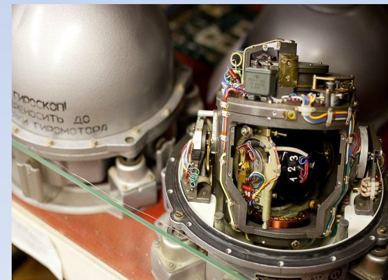
Авиационный гироскоп
