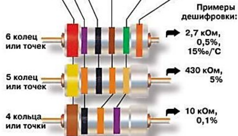
Рис. 3.2. – Маркировка параметров резисторов с помощью цветных полосок.
