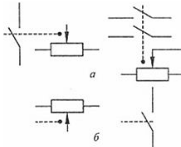
УГО переменных резисторов, объединенных с выключателем.
