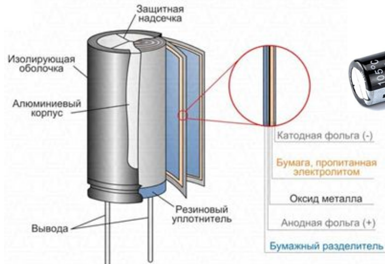
Конструкция радиального электролитического конденсатора
