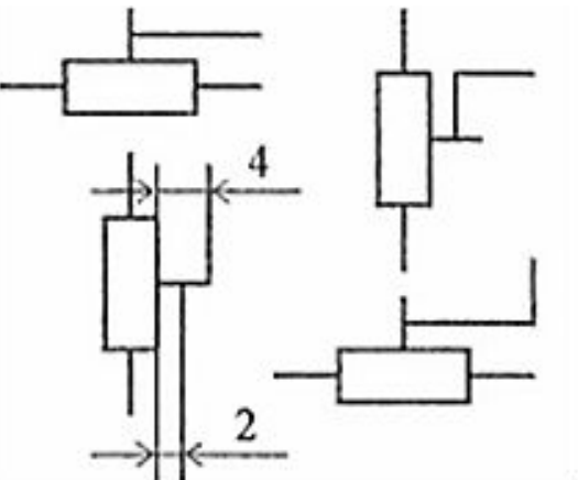
УГО подстроечного резистора.
