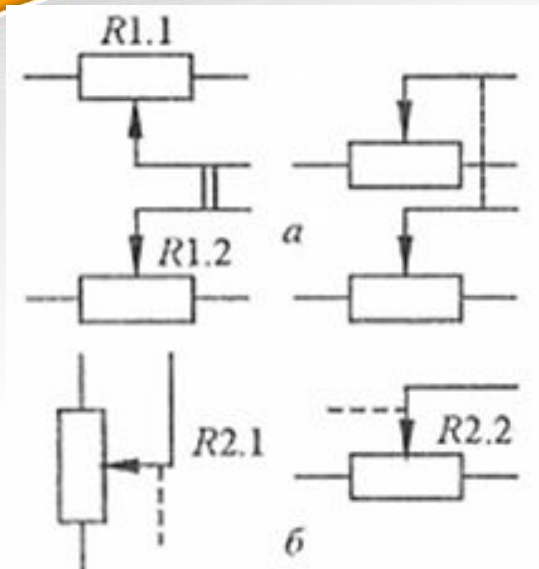
УГО сдвоенных переменных резисторов.
