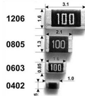
Миниатюрные резисторы.
