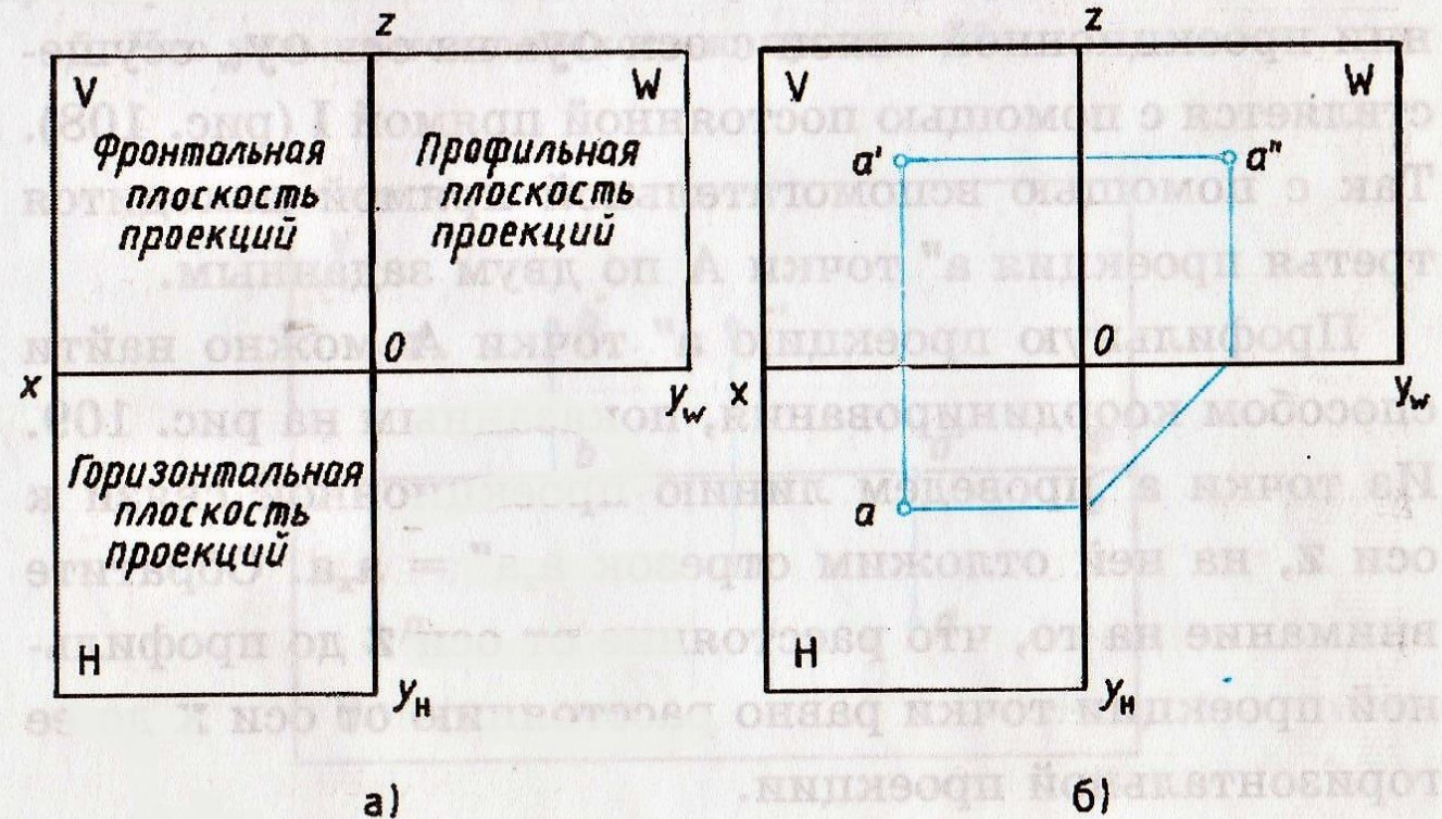
Чертеж точки в системе прямоугольных проекций
