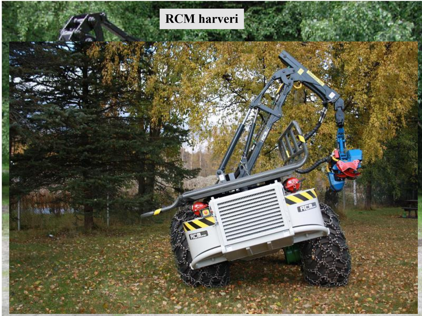
Kuva 4. Harveri-pienharvesteri (Kuva: Artekno Oy).
