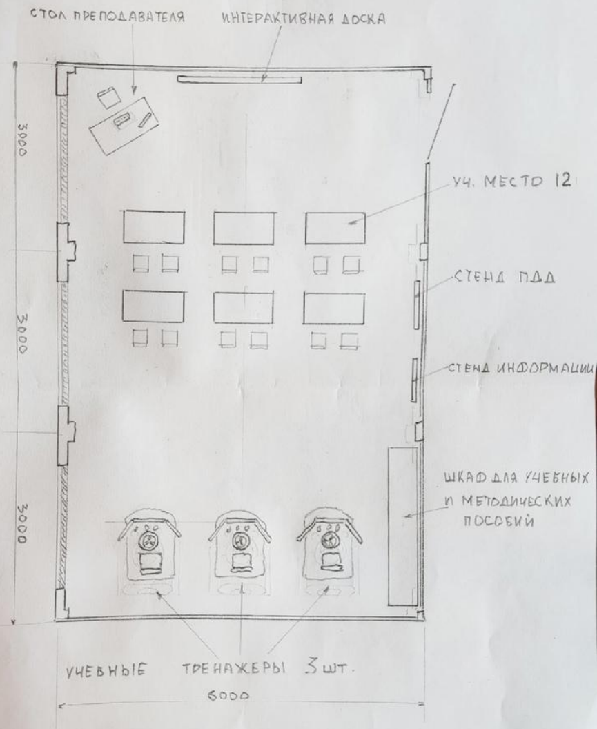
ПЛАН АВТОКЛАССА «УЧИМСЯ ВОДИТЬ»
