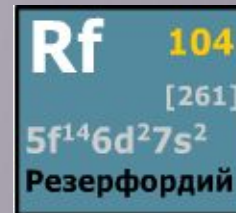
104 элемент Периодической системы Менделеева
