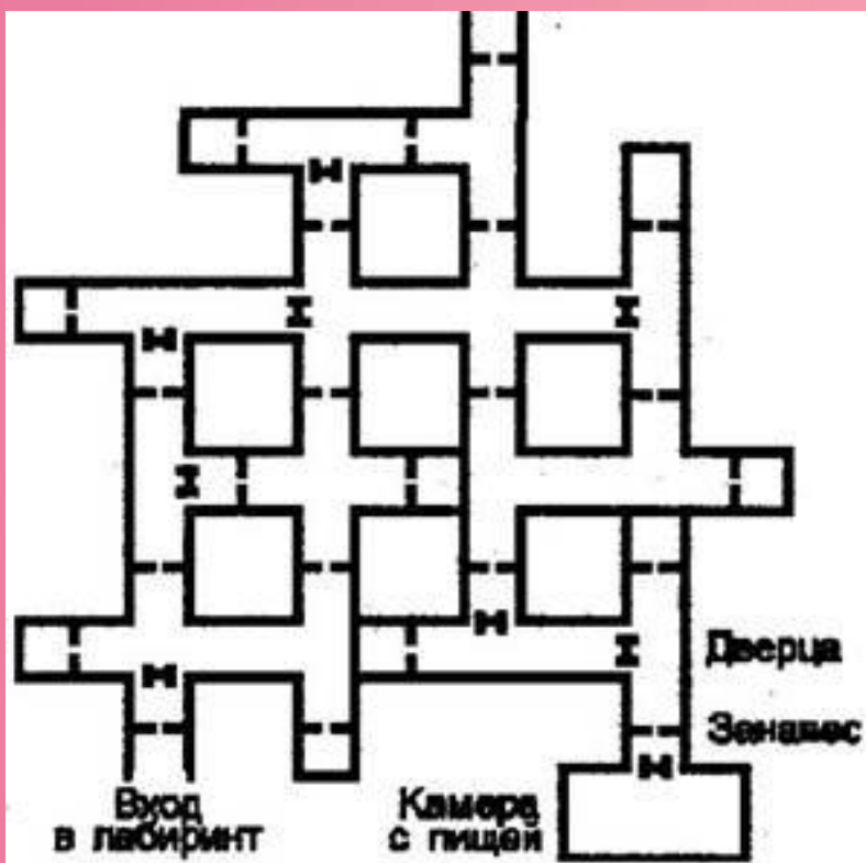
Рис. 4. Схема лабиринта с 14 Т-образными коридорами (по Эллиоту, 1928)
