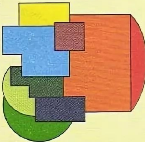
Многоядерная модель
