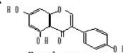
Изофлавоны
