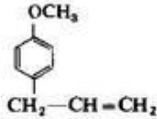
Метилхавивол (эстрагол)
