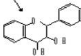
Лейкоантоцианидины
