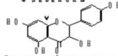
Дигидрофлавонолы
