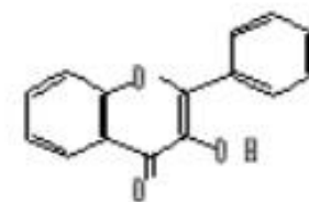
Флавонолы
