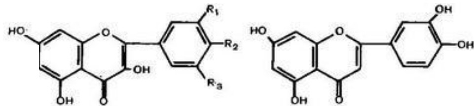
R 1 R 2 R 3 Комферол H OH H Навреттин OH OH H
