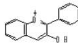
Антоцианидины
