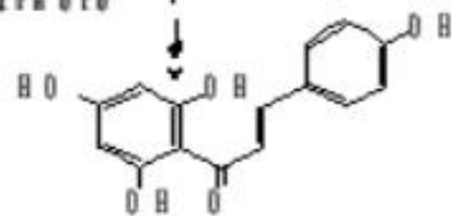
Халконы
