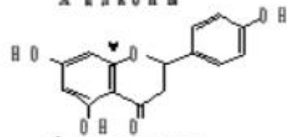
Флаваноны
