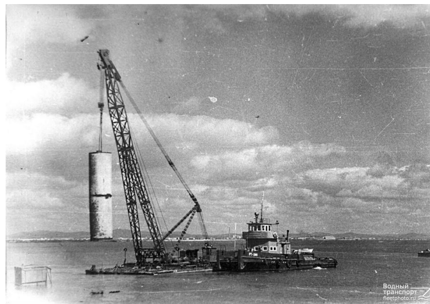
Плавучий кран ПРК – 30/50
