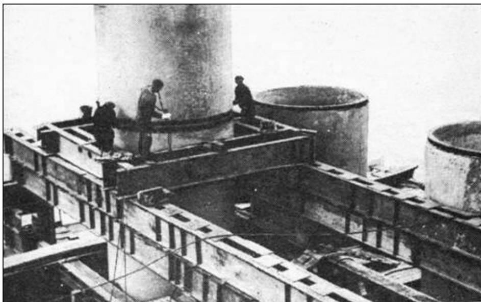
Установка железобетонных оболочек в направляющий каркас
