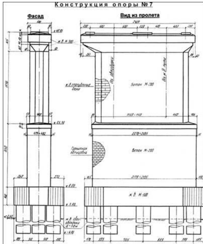
Схема промежуточной опоры моста у г. Комсомольск-на-Амуре.
