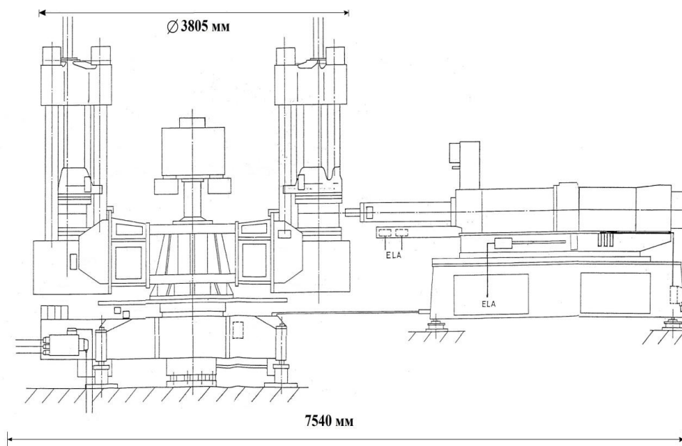
Рис. 3 - машина «Десма» и её вид в разрезе
