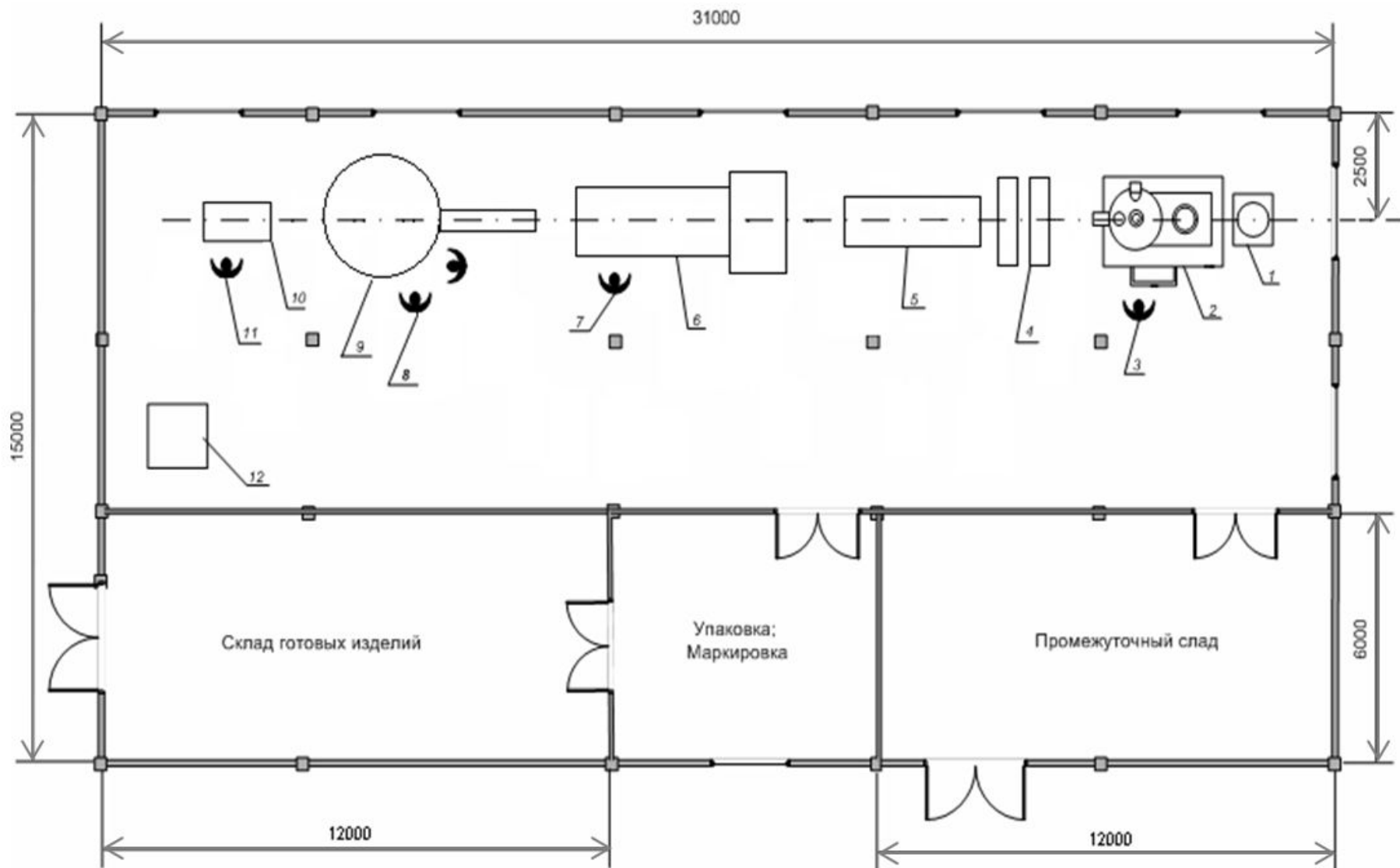
План участка производства резиновых шапочек
