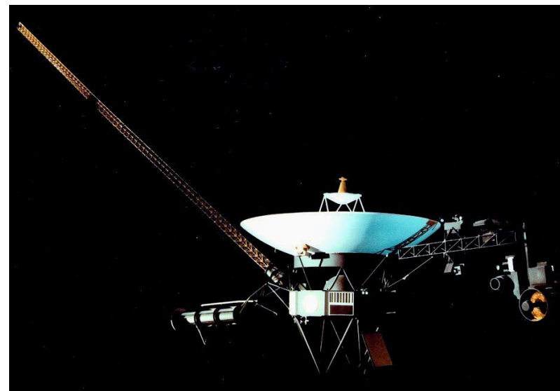
«Вояджер-2»
