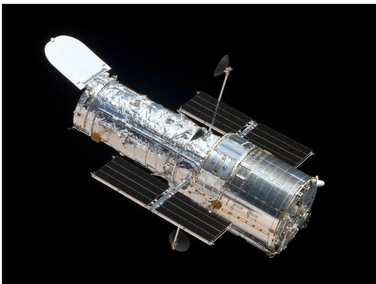
телескоп «Хаббл»
