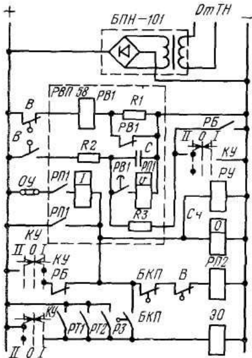
Схема АПВ карьерной линии
