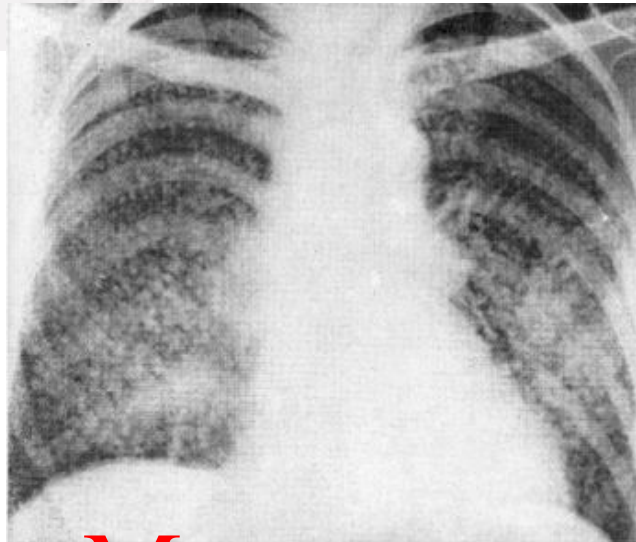
Метастазы
