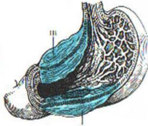
Эндофитный рост
