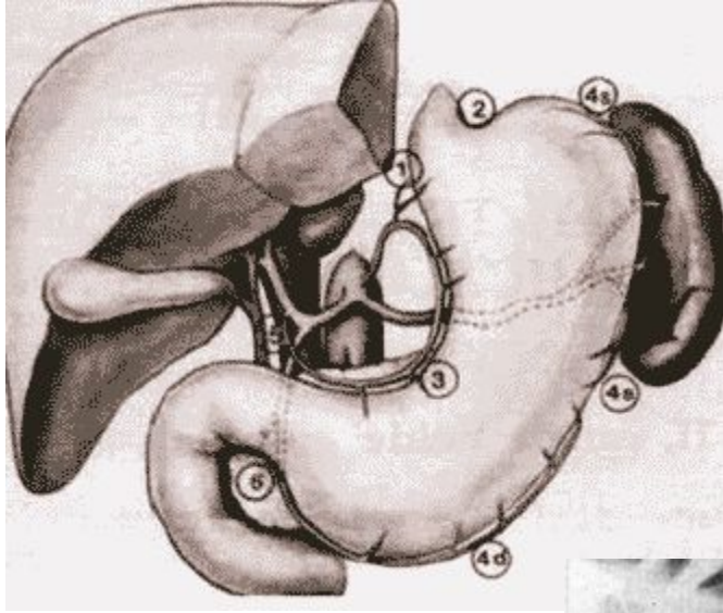
Региональные лимфоузлы
