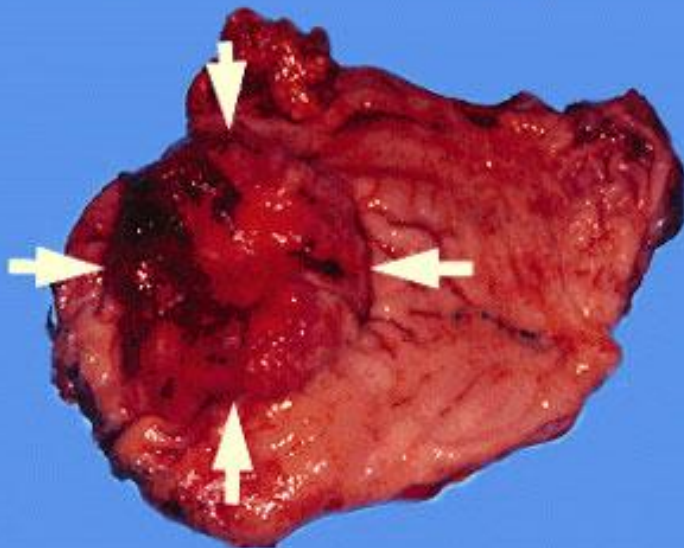
Аденокарцинома желудка
