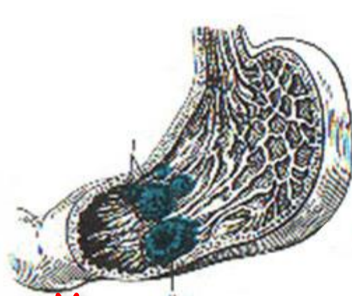
Экзофитный рост
