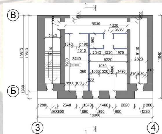
Обмерный план мансарды
