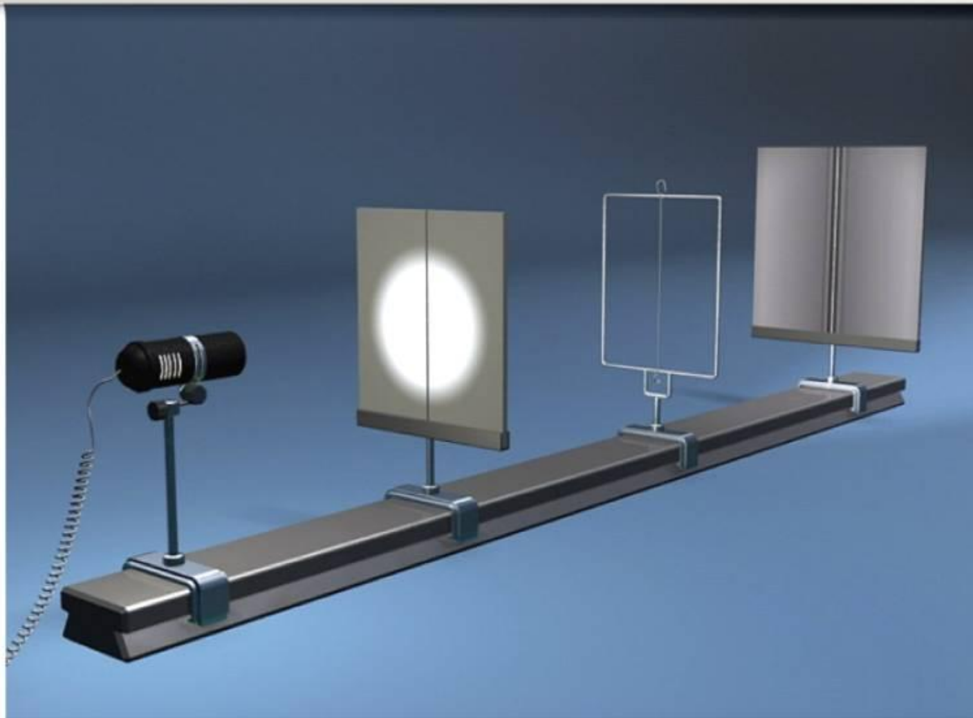
Опыт по наблюдению дифракции от тонкой нити (часть 2).
