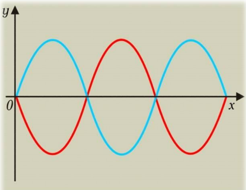
Условие минимумов.
