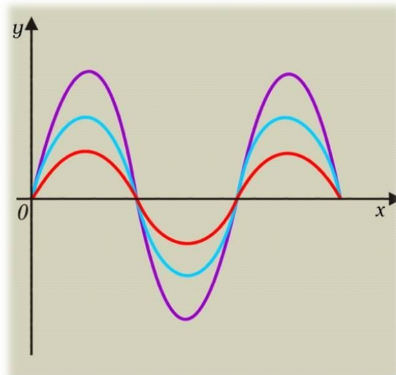
Условие максимума.
