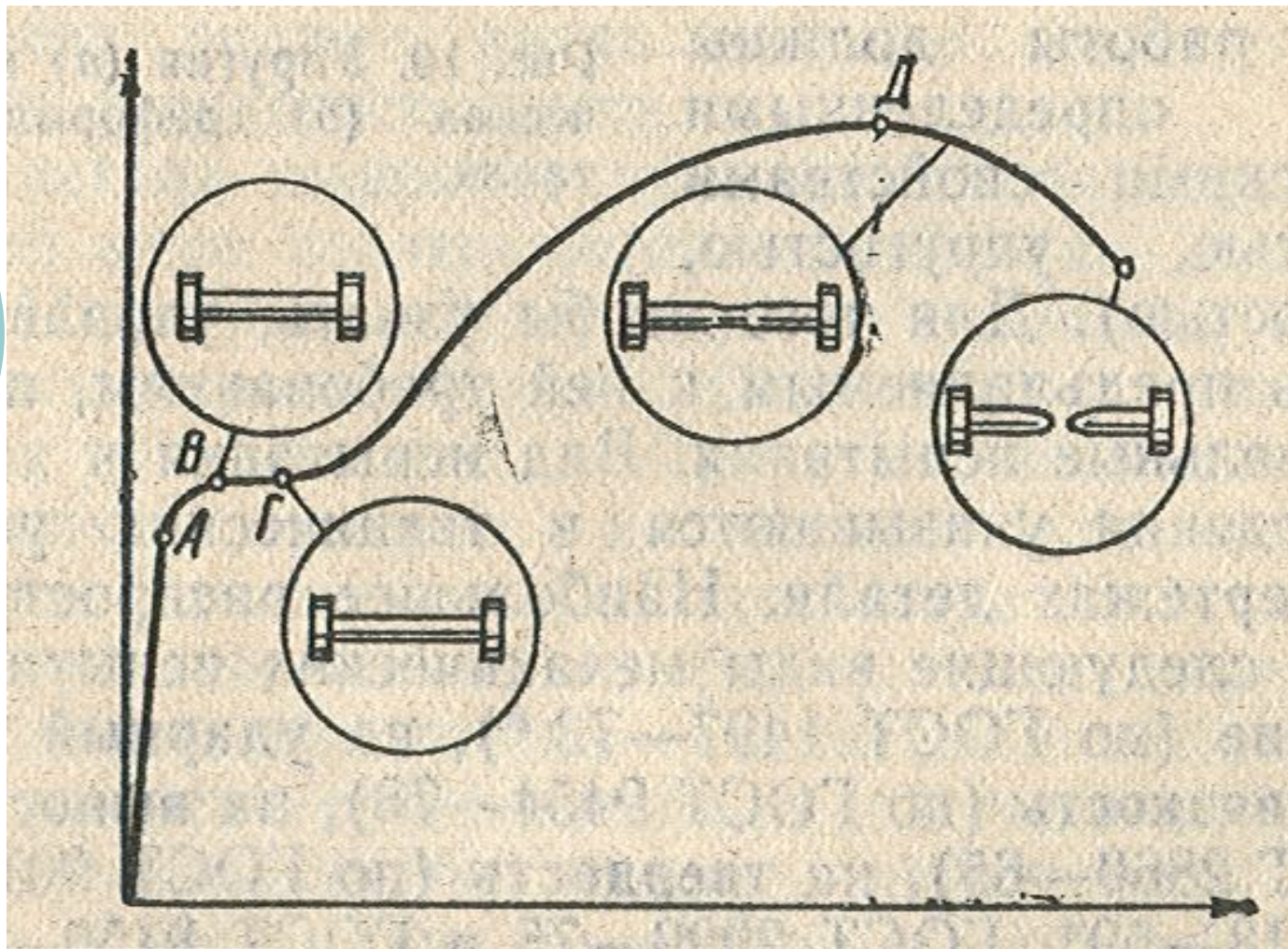
Диаграмма растяжения стального образца.
