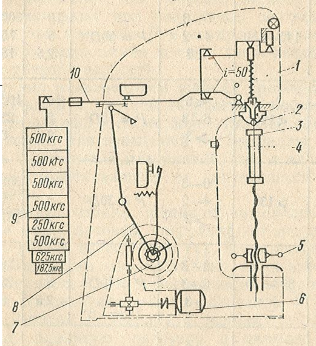
Схема прибора Бринелля.
