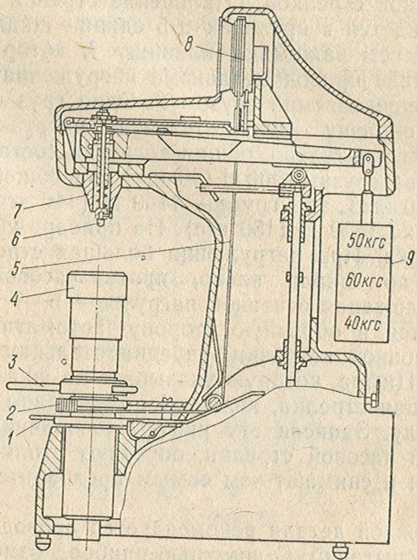
Схема прибора Роквелла.
