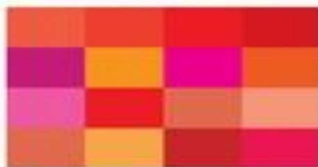
Изохромная
