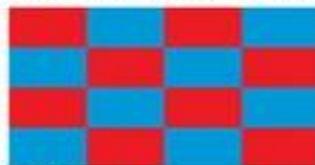
Полярная
