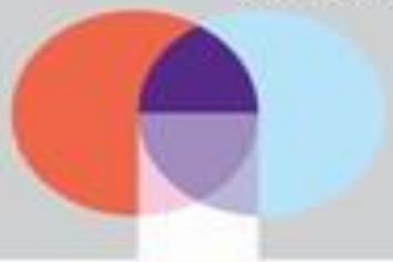
Изменение насыщенности
