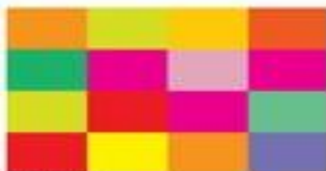
Мерохромная
