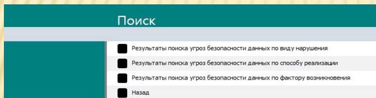
Рисунок 3 - Поиск
