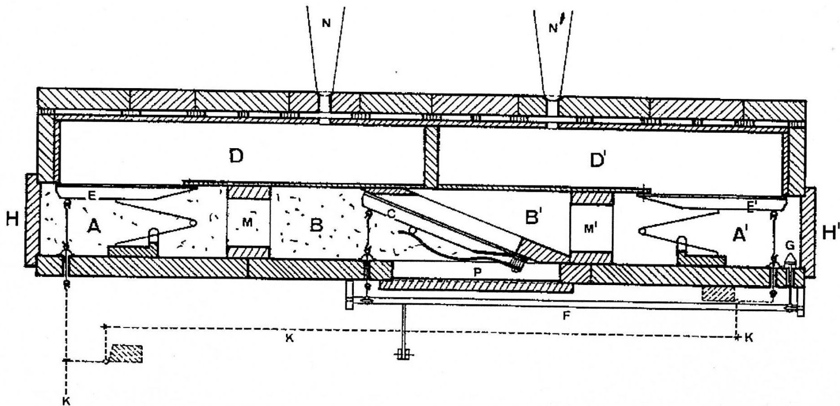
Двойная виндлада (система, применённая Аристидом Кавайе-Коллем в органах, в том числе в органе Большого зала Московской консерватории).
