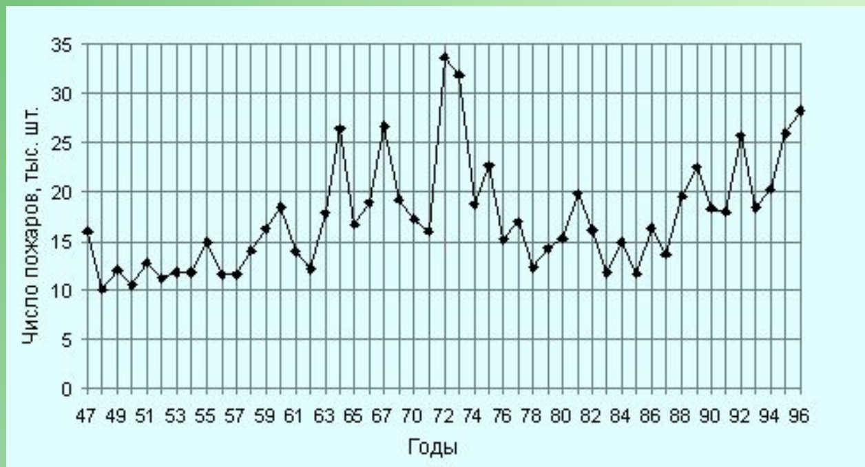
Рис. 1. Динамика числа лесных пожаров на охраняемой территории России в 1947-1996 годах.
