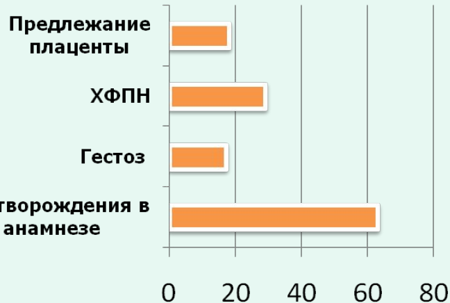
Курганский областной перинатальный центр 100 историй родов
