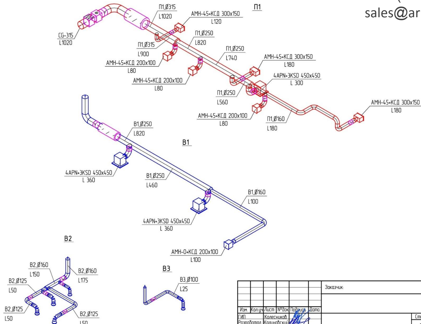
АксонOMETрическая схема системы вентиляции
