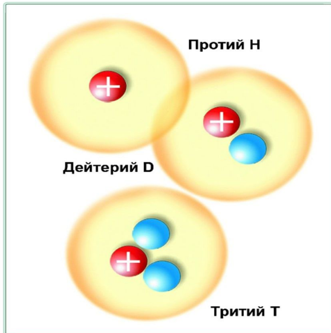
Изотопы водорода
