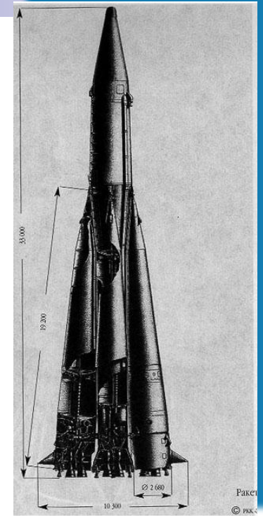
Ракета Р-7
