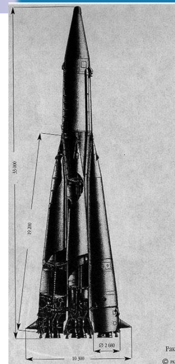
Ракета Р-7
