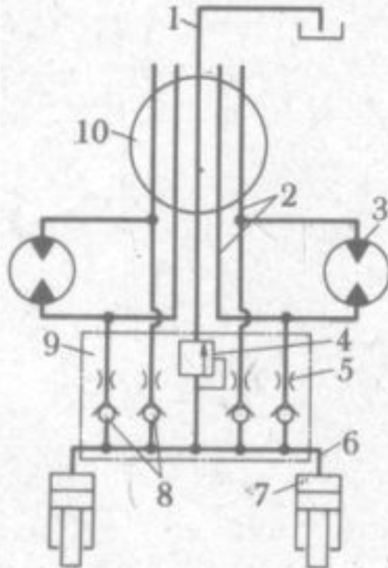
Рис. 6 Схема гідросистеми натягу гусениць 1, 2, 6 – трубопроводи; 3 – гідромотор; 4, 8 – клапани; 5 – дросель; 7 – гідроциліндр; 9 – блок клапанів; 10 - колектор
