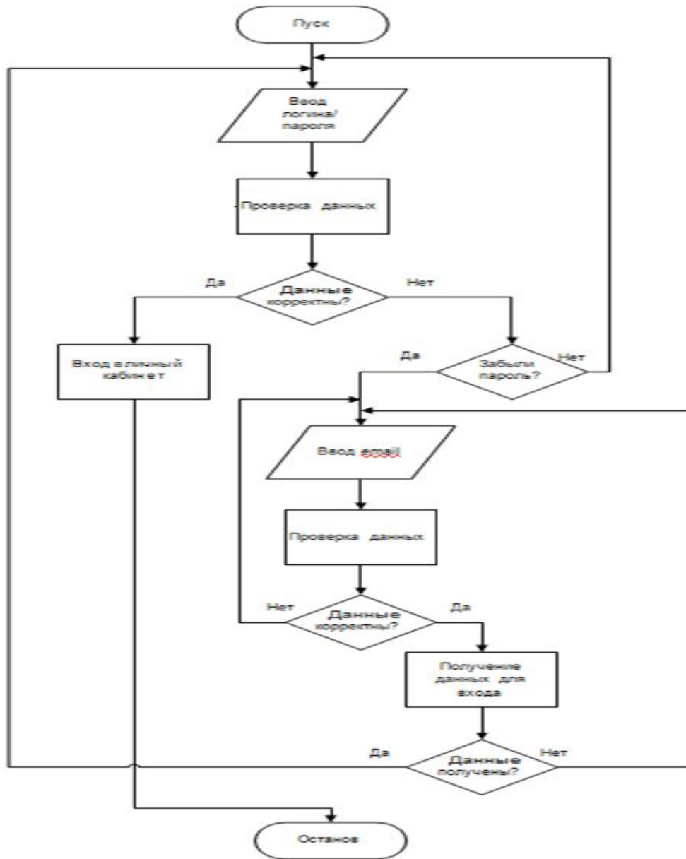
Алгоритм входа в личный кабинет пользователя
