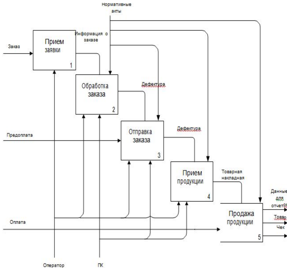
Диаграмма «Оказание услуги клиенту»
