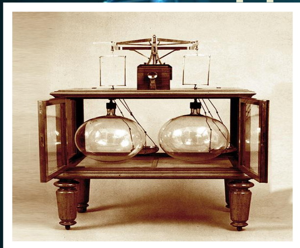
Весы для взвешивания газообразных веществ
