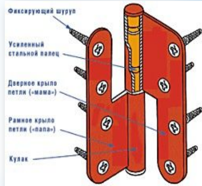
Петля в разрезе
