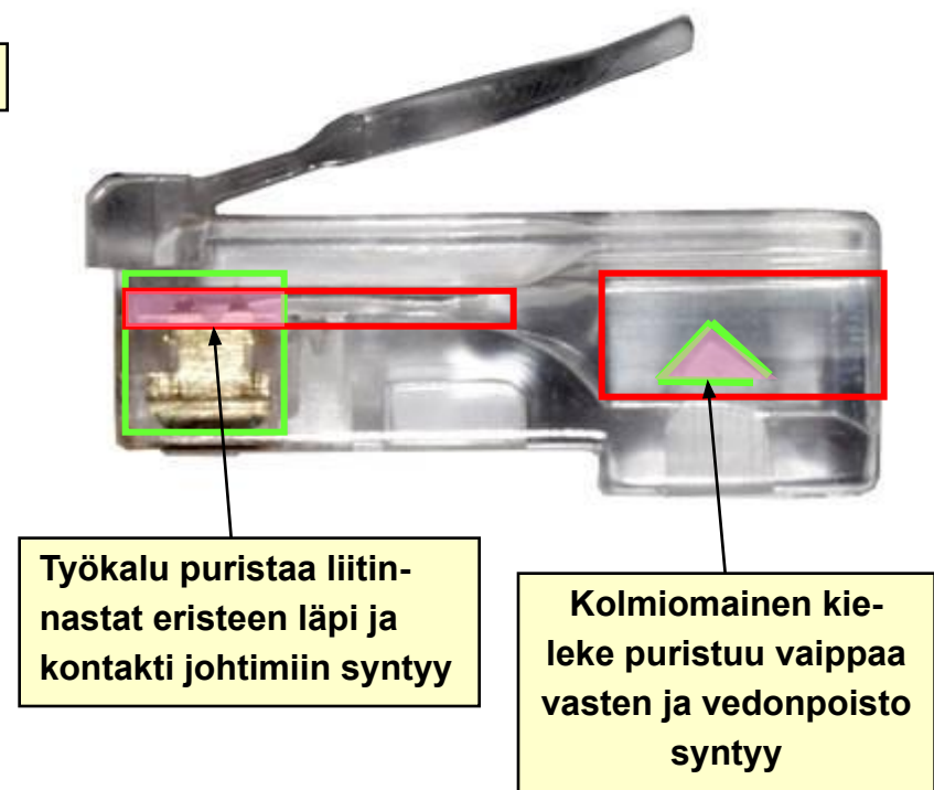
Puristettu liitin
