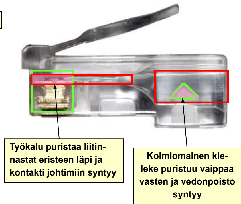
Puristettu liitin
