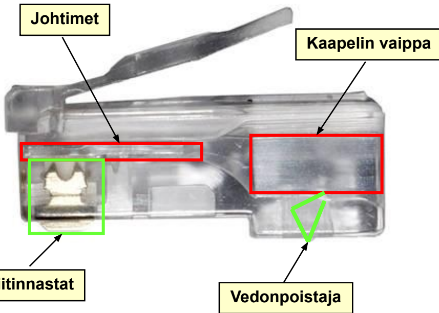
Ei-puristettu liitin
