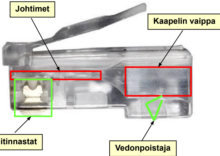
Ei-puristettu liitin
