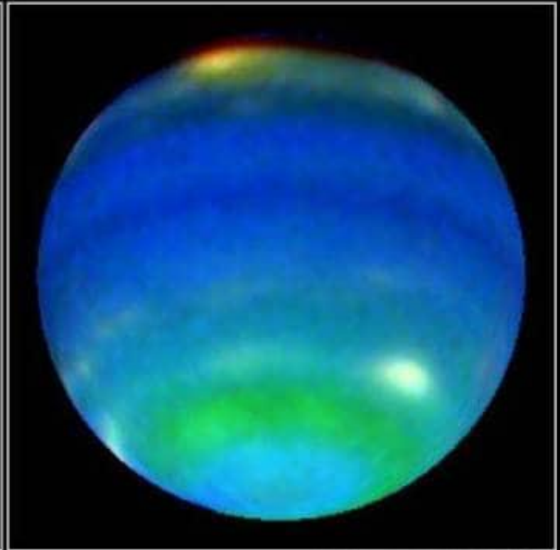
HST · WFPC2
