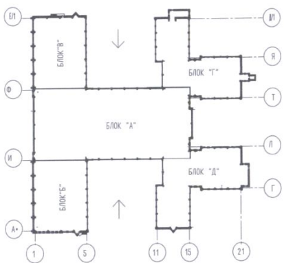
СХЕМАТИЧЕСКИЙ ПЛАН
