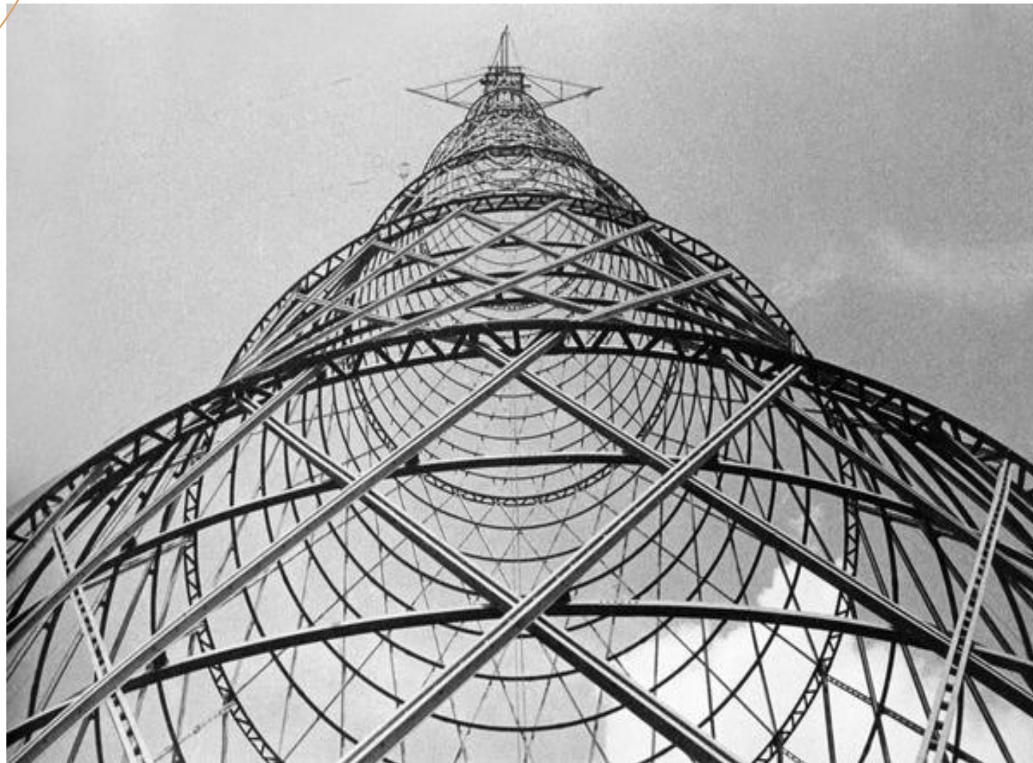
«Шуховская башня», 1920
