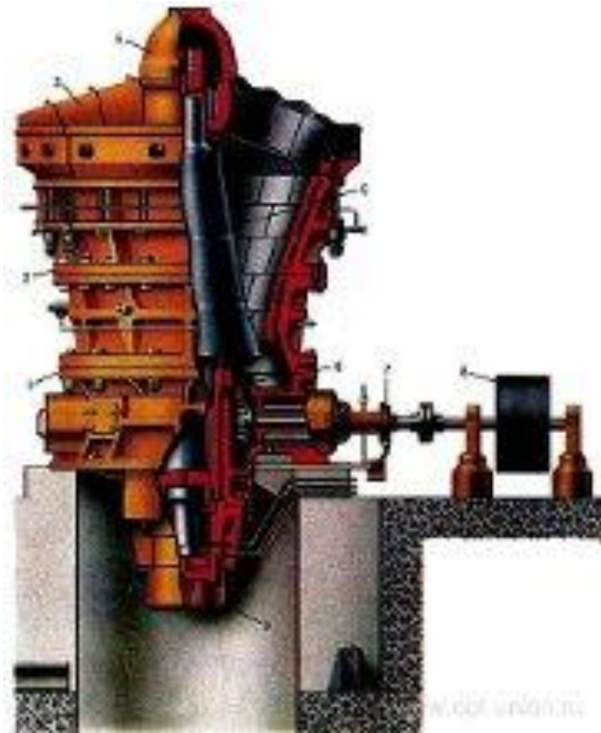
Конусная дробилка
