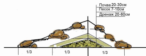
Схема устройства альпийской горки
